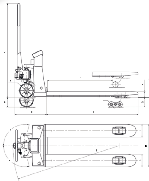
Transpalette ARXLCD Wide (pour palettes américaines)
