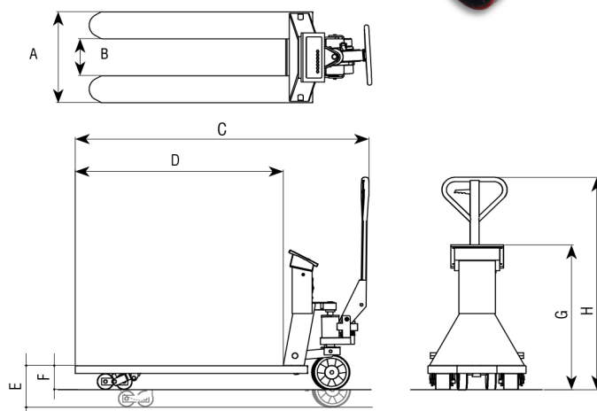
Transpalette TP410 Wide (pour palettes américaines)
